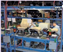
NHKシーティングオブアメリカの自動車用シート組立てライン
